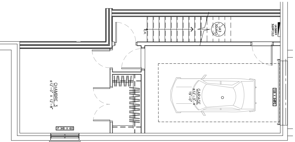
PLAN SOUS-SOL
