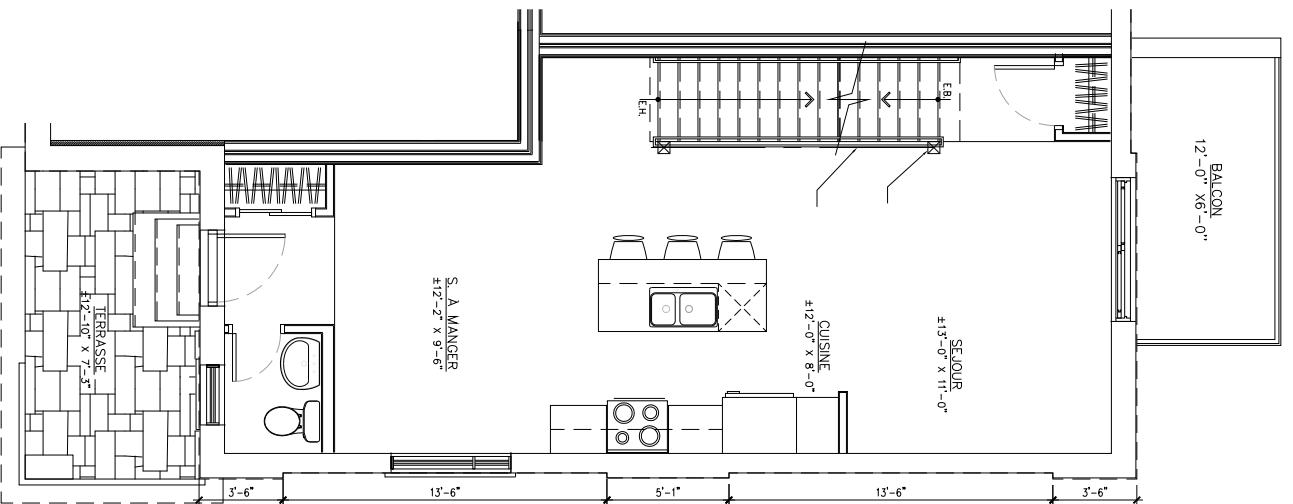
PLAN R.D.C.
