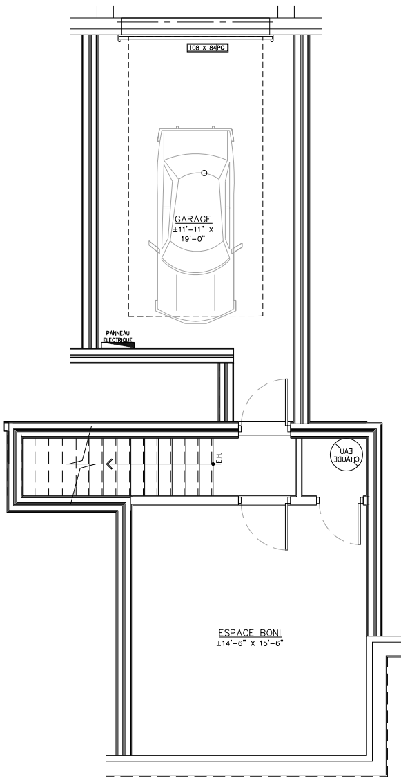
PLAN SOUS-SOL
