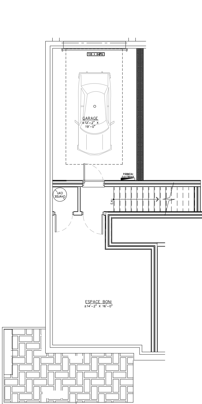
PLAN SOUS-SOL
