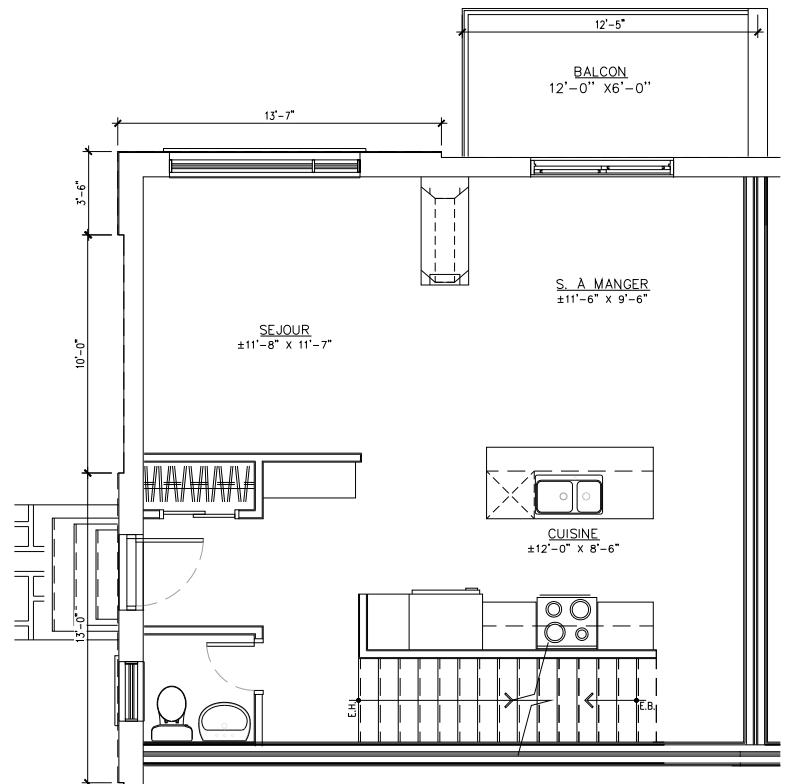
PLAN R.D.C.
