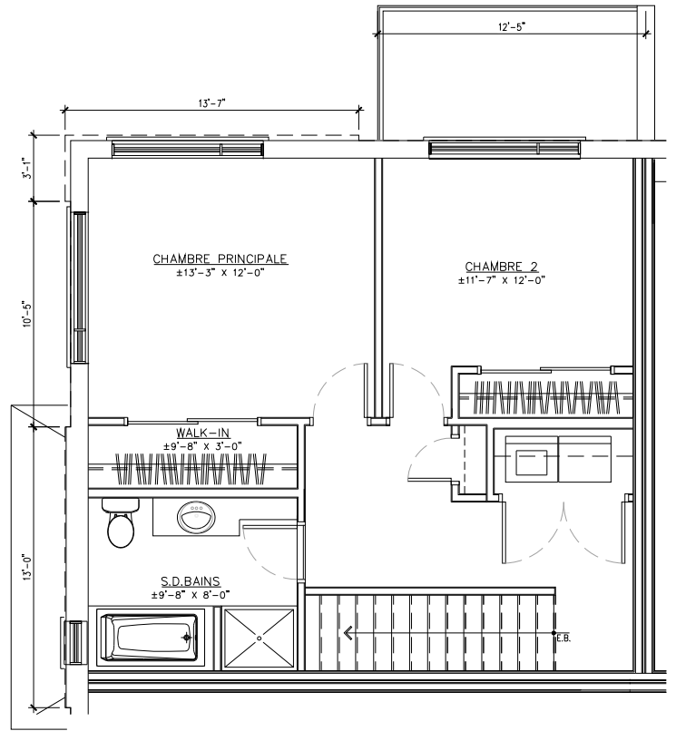
PLAN ÉTAGE
